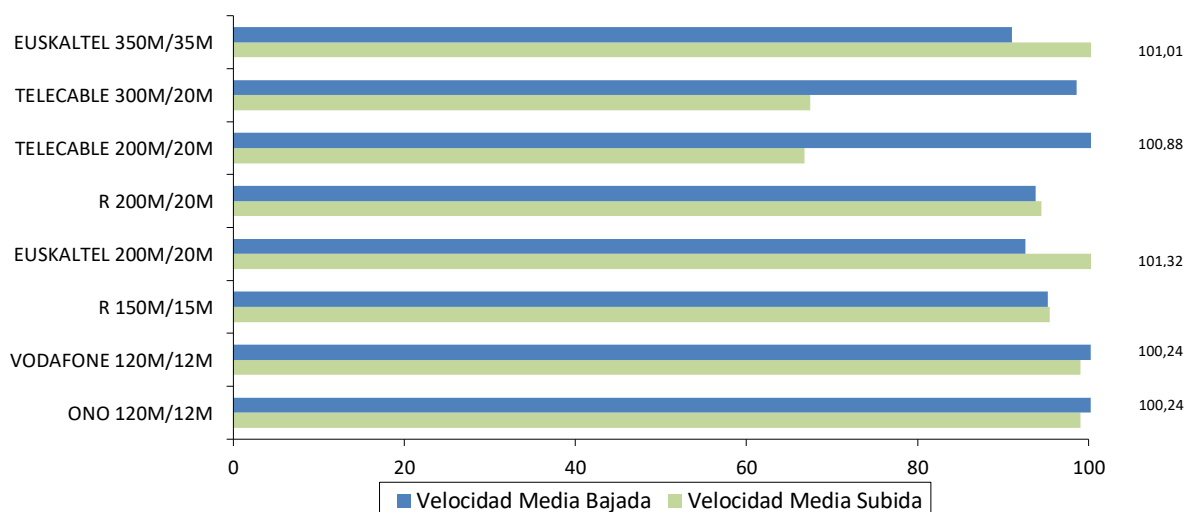
Velocidad nominal superior a 120 Mbps Porcentaje sobre la velocidad nominal (%)
